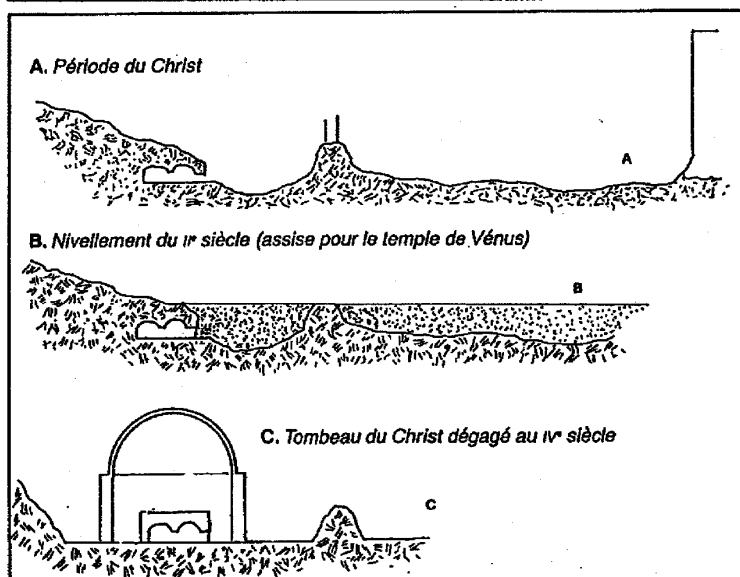
Coupe du terrain sous le Calvaire et l'Anastasis
