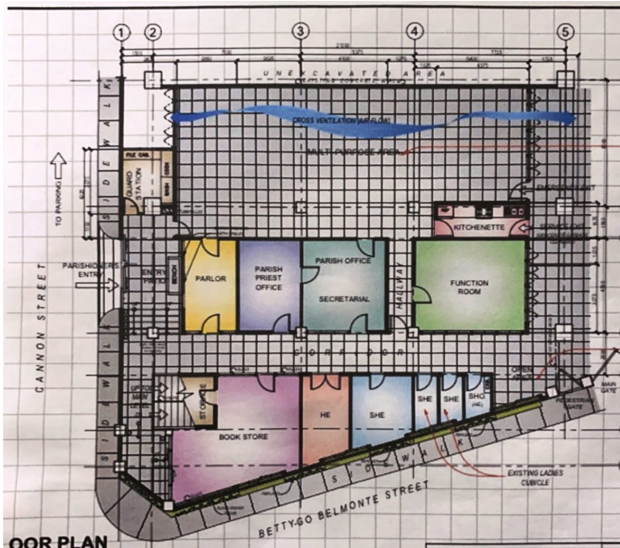
Le plan du sous- sol, dessiné par l'architecte
