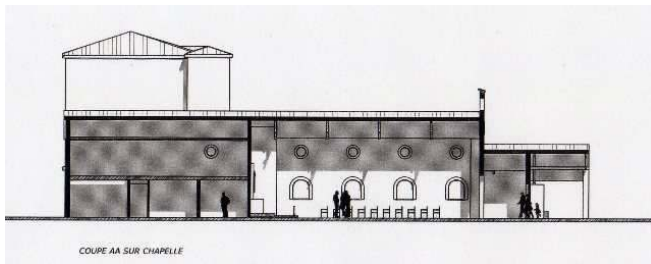
bureaux-sacristie / chapelle / préau Coupe latérale du nouveau bâtiment
