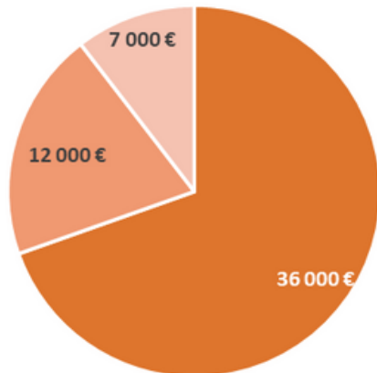
Dépenses
